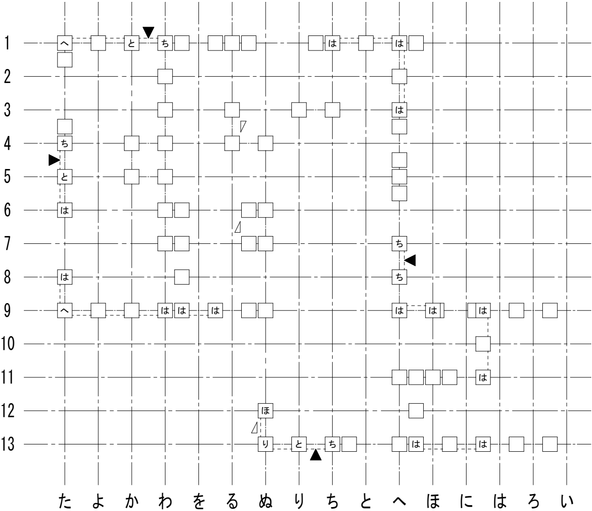
1 階柱壁伏図
